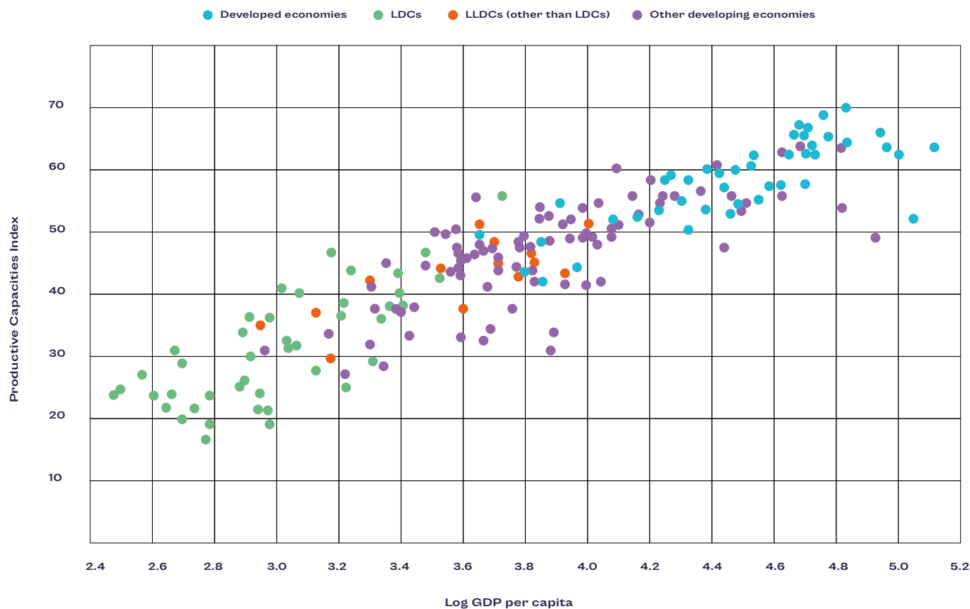
2. grafikoa. Produkzio-ahalmenaren indizearen (KSIaren) eta per capita BPGaren arteko korrelazioa (2020-2022)
